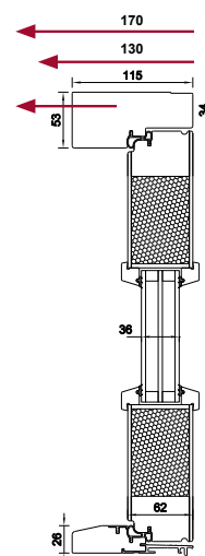
DURVJU KĀRBAS BIEZUMA PAPLATINĀJUMI
