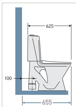
UZ GRĪDAS LIEKAMĀIS PODS
