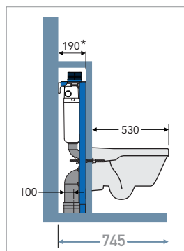
AIZSTĀTS AR PIEKARAMO PODU UN TRIOMONT IEBŪVĒJAMO RĀMI
