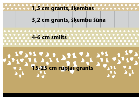
Lai izturētu vieglo automašīnu slodzes, tiek sagatavota 15-25 cm rupjas grants pamatne, uz kuras tiek uzbūvēts un sablīvēts 4-6 cm smilts slānis.
